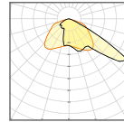
Lichtverteilung ASYM 50° x 110°
