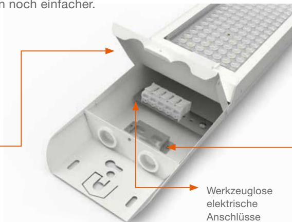
Werkzeugloses Öffnen/Schließen der im Lieferumfang enthaltenen Endkappen für Zugang zu elektrischen Anschlüssen
