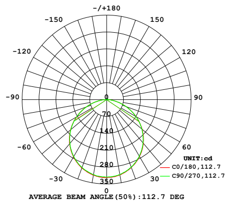
65792, 10W
