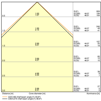
LN INV DI 1500 P 69W 930 EM WT LN INV DI 1500 P 69W 930 PS EL WT 1400mA
