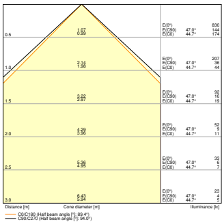
LN INV DI 1500 P 69W 940 DAVR EM BK LN INV DI 1500 P 69W 940 DA EL BK 1400mA
