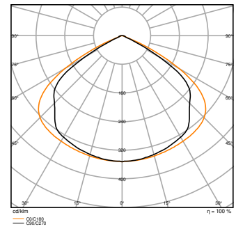
LB FLEX 1500 P 140W 840 VW
