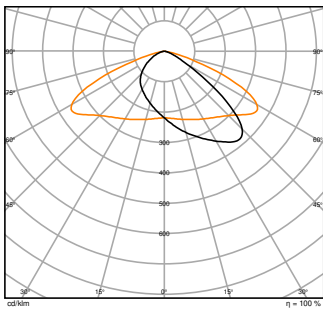
FL PFM DA 290W 3000K ASYM 45X140 BK
