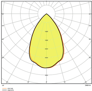
LDPFM DL G2S 190 3500lm 700mA 865
