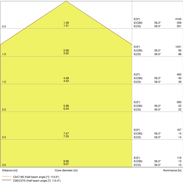
PL PFM 625 25W 4000K LDT
