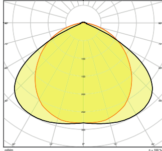
TRUSYS PFM 50W 4000K VW
