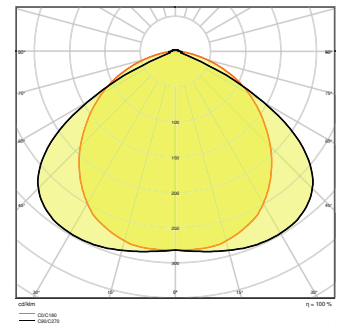
TRUSYS PFM 50W 4000K VW
