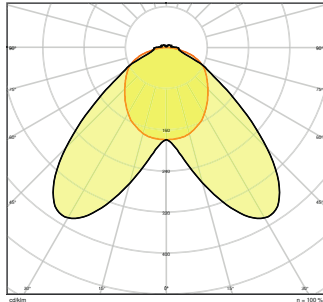
TRUSYS PFM 35W 4000K DS
