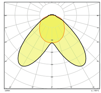
TRUSYS PFM 50W 4000K DS 4x1 EUE LEDV
