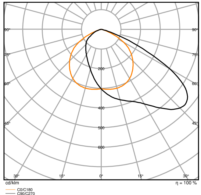
FL PFM 50W 3000K ASYM 55X110 BK
