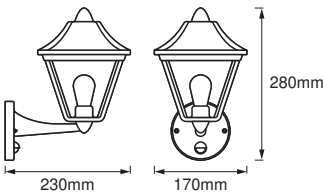
ENDURA CLASSIC TRAD UPSENS ALU E27 GD
