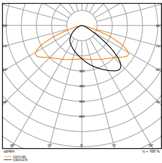
FL PFM DA 290W 3000K ASYM 45X140 BK
