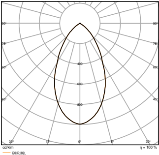
DL CMFT DA D250 P 42W MS 940 U19 WT
