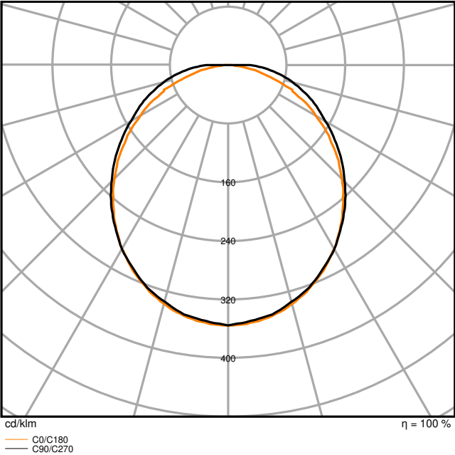
LN SF 1500 ZB P 45W 830 WT IP44
