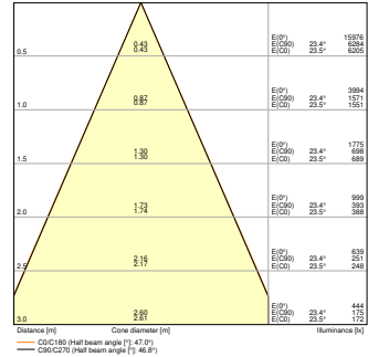
TR SP XR V 20W 930 WT 50D
