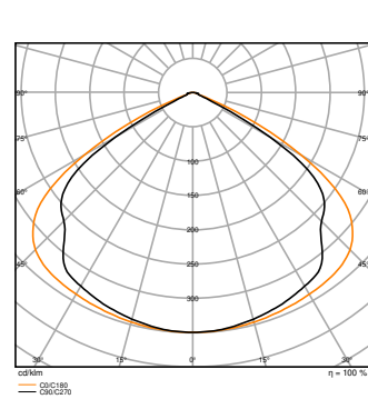
LB FLEX 1500 P 73W 840 VW
