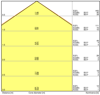
PL CMFT 625 P 33W 840 ZBVR EM CONVERSION BOX
