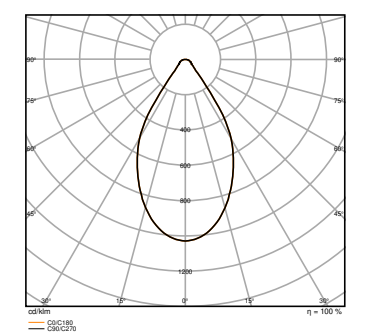
HB DA P 200W 840 70DEG IP66
