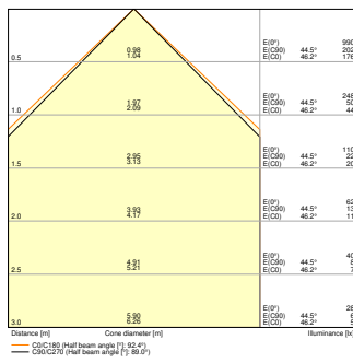
LN INV DI 1500 P 69W 940 DAVR EM WT
