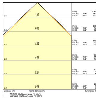
LN INV DI 1500 P 69W 940 DA EL WT 1400mA
