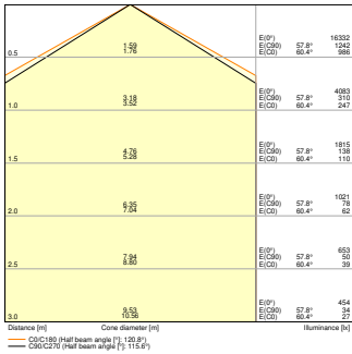
LB FLEX 1500 P 73W 840 VW
