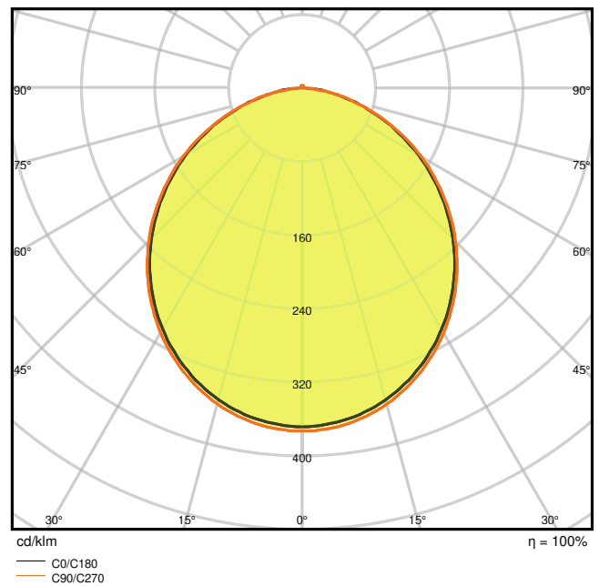
4058075052543 DL SLIM SQ155 12W 4000K WT IP20
