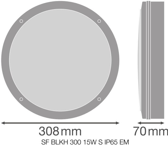
SF BLKH 300 15W S IP65 EM
