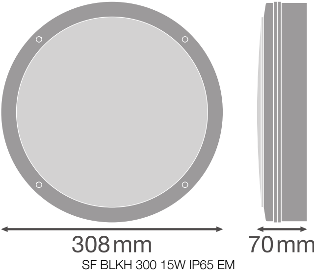
SF BLKH 300 15W IP65 EM
